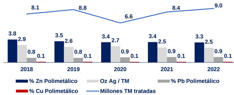
Gráfico 6: Evolución de la producción y leyes promedio
